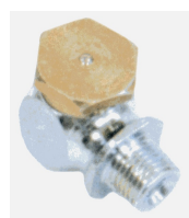
INGRASSATORE TIPO R66 FILETTO GAS. Gambo di montaggio esagonale con chiave mm. 14 testa piatta esagonale mm. 15 smontabile sul 90 gradi.
